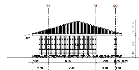
E3000 Alçado Lateral Esquerdo Left Side Elevation
