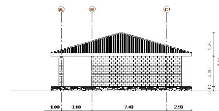
E3000 Alçado Lateral Direito Right Side Elevation
