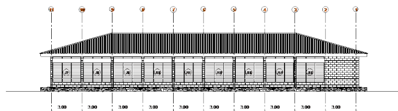
E3000 Alçado Posterior Back Elevation
